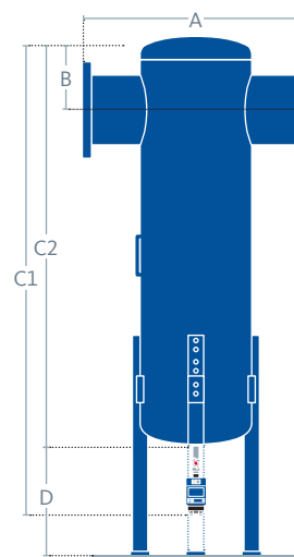
Filtros con brida (L080 – L304)
